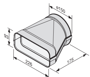
DFK-A • Adapter flad – rund M.-nr. 10811430 Pris kr. 275,00
