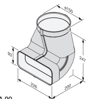
DFK-A 90 • Adapter flad – rund 90° M.-nr. 10811440 Pris kr. 275,00
