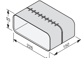
DFK-L • Ved pladsmangel (hvor DFK-V ikke kan bruges) • Ved montering sættes forlængerstykket DFK-L på fladkanalstykket, fladkanalen monteres, og forlængerstykket DFK-L skubbes over samlingen M.-nr. 11051270 Pris kr. 275,00
