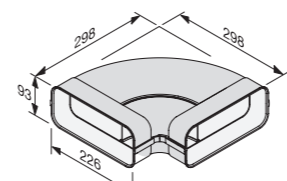
DFK-BH 90 • Horizontal bue 90° M.-nr. 10811390 Pris kr. 275,00
