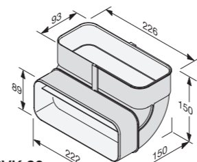
DFK-BVK 90 • Vertikal bue 90° • 150 mm dyb og høj M.-nr. 10811470 Pris kr. 275,00
