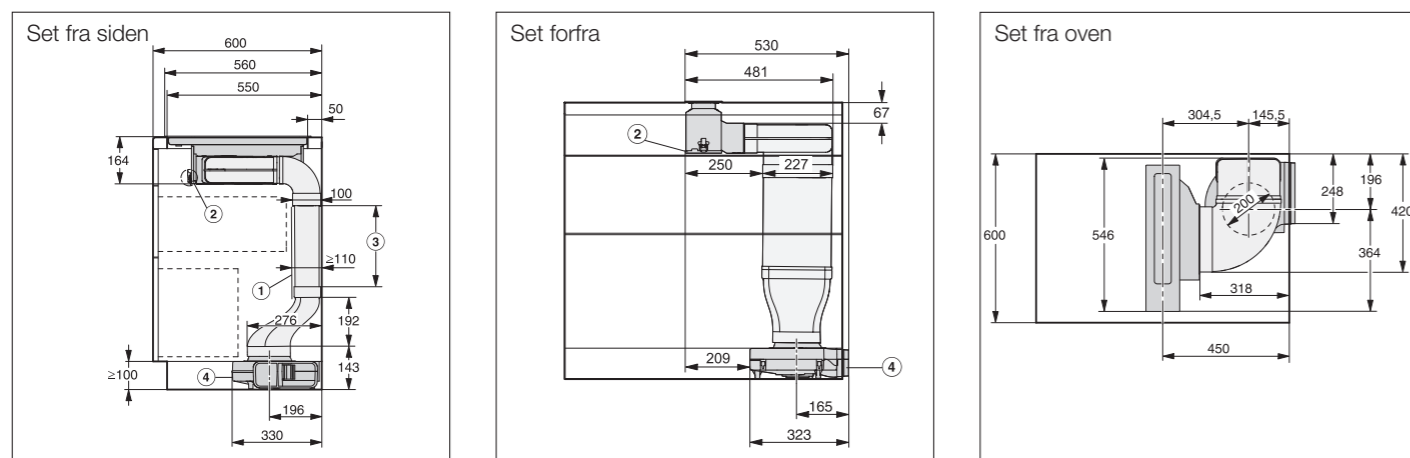
CSDA 7000 FL – luftkanal til højre, planforsænket i 600 mm dyb bordplade
