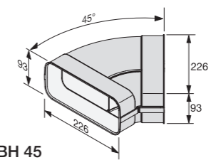
DFK-BH 45 • Horizontal bue 45° M.-nr. 10811450 Pris kr. 275,00
