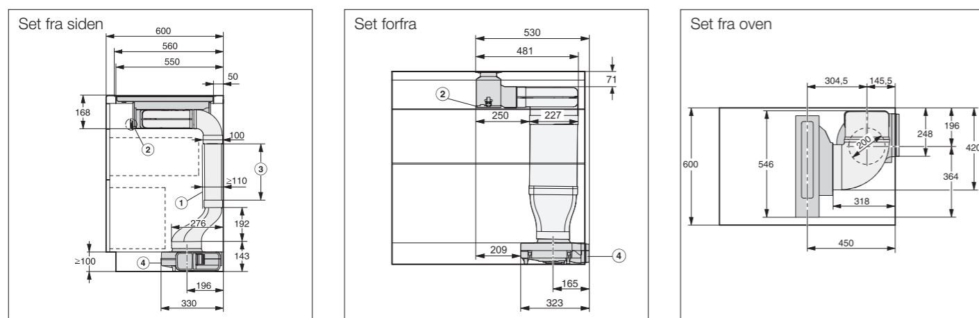
CSDA 7000 FL – luftkanal til højre, monteret oven på >600 mm dyb bordplade
