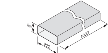
DFK-R 1000 • Lige stykke, 1 m M.-nr. 10811340 Pris kr. 275,00
